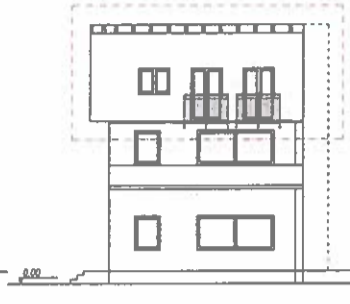
Ansicht Westen
